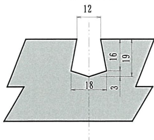
目地部詳細
