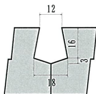
目地部詳細
