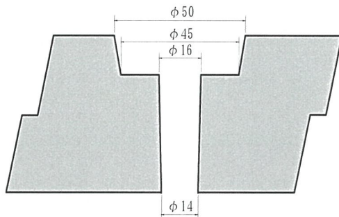
穴部分 詳細
