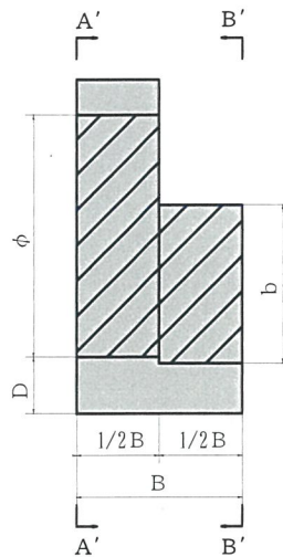
側面図
