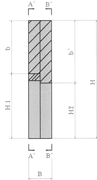
側面図
