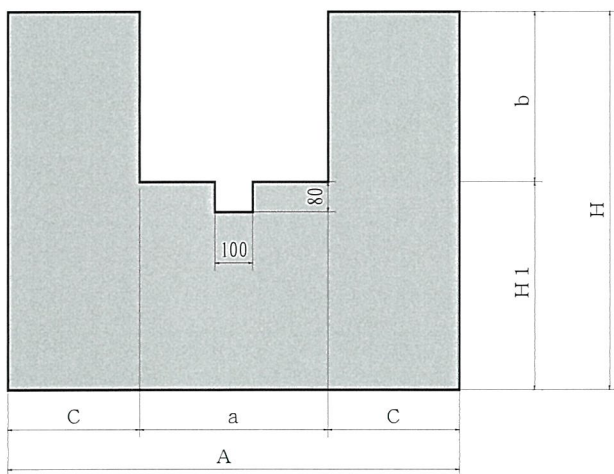
規格寸法表
