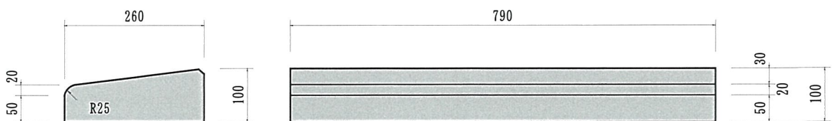
特殊B変形 260×100×790 参考重量 37kg
