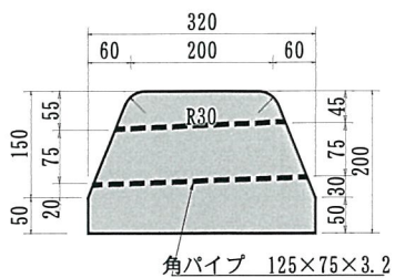
Ⅳ型縁石（箱抜）
