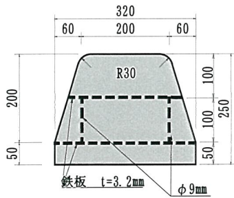
Ⅲ型縁石（スクリーン）
