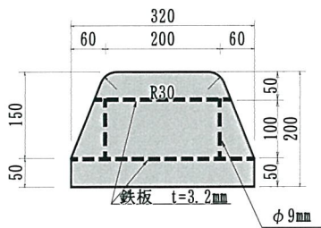
Ⅳ型縁石（スクリーン）
