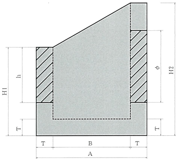
規格寸法表
