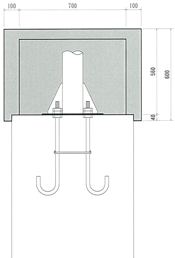
正面図
