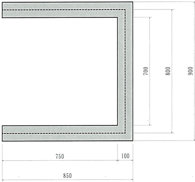
側面図
